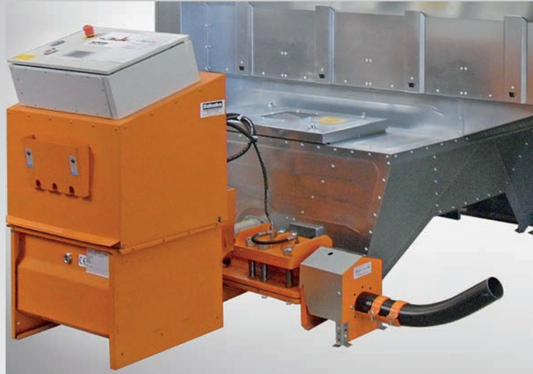
Beispiel: Spänebehälter SPB 100/4/130 an VACOMAT mit einer Brikettierpresse Compacto
